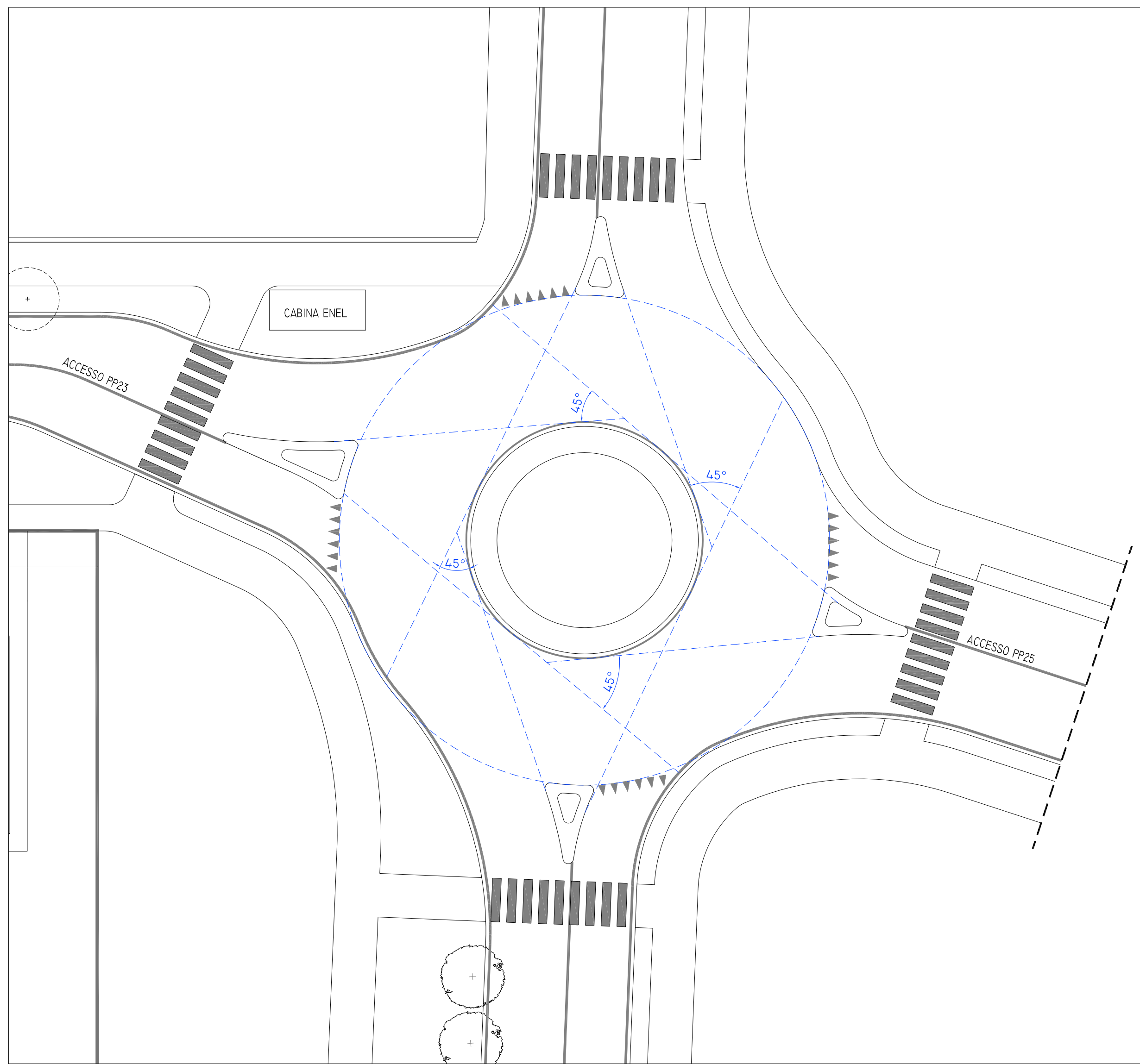
PLANIMETRIA SCALA 1:200 ⊕ VERIFICA ANGOLO DI DEVIAZIONE - DM 19/04/2006
