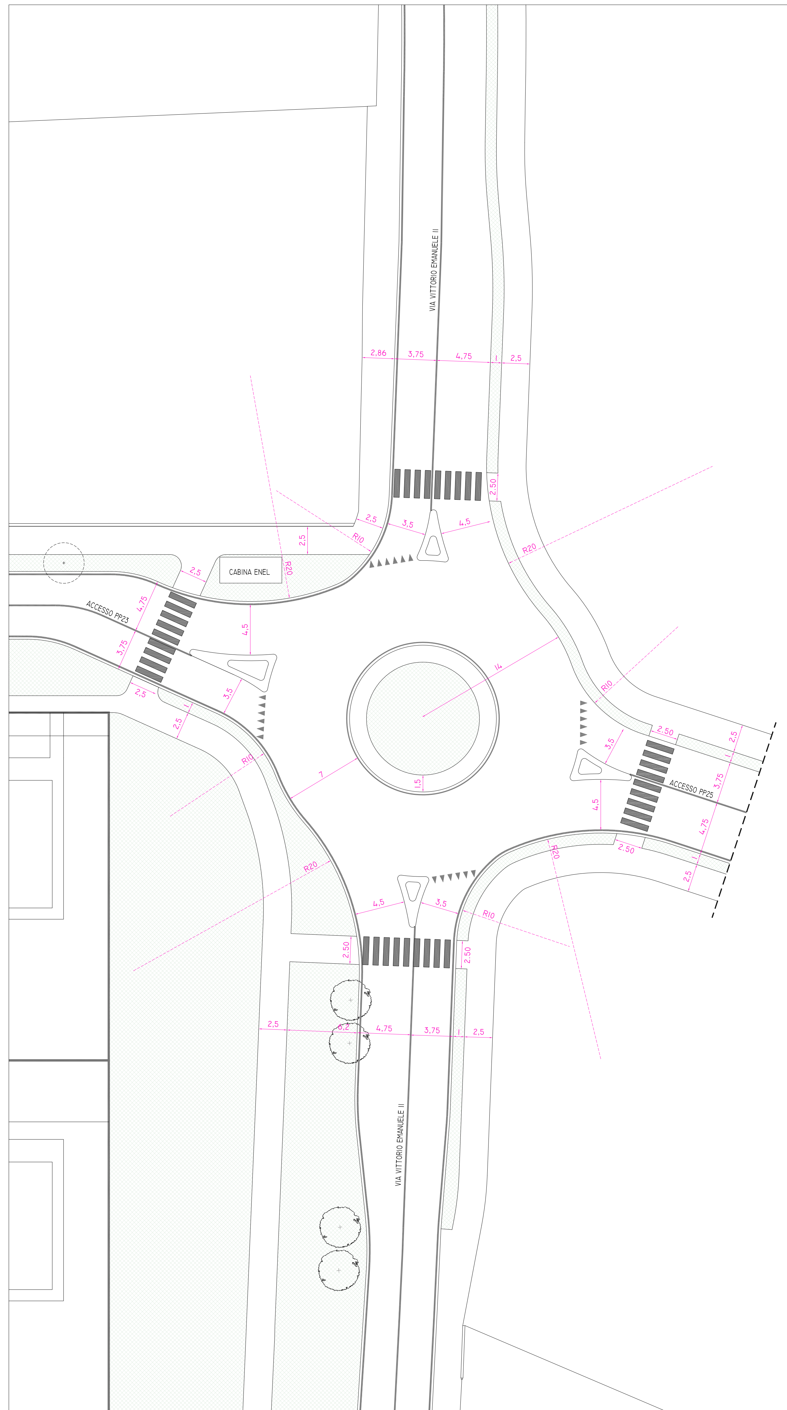
PLANIMETRIA SCALA 1:200 ⊕ PROGETTO INTERSEZIONE A ROTATORIA AI SENSI DM 19/04/2006
