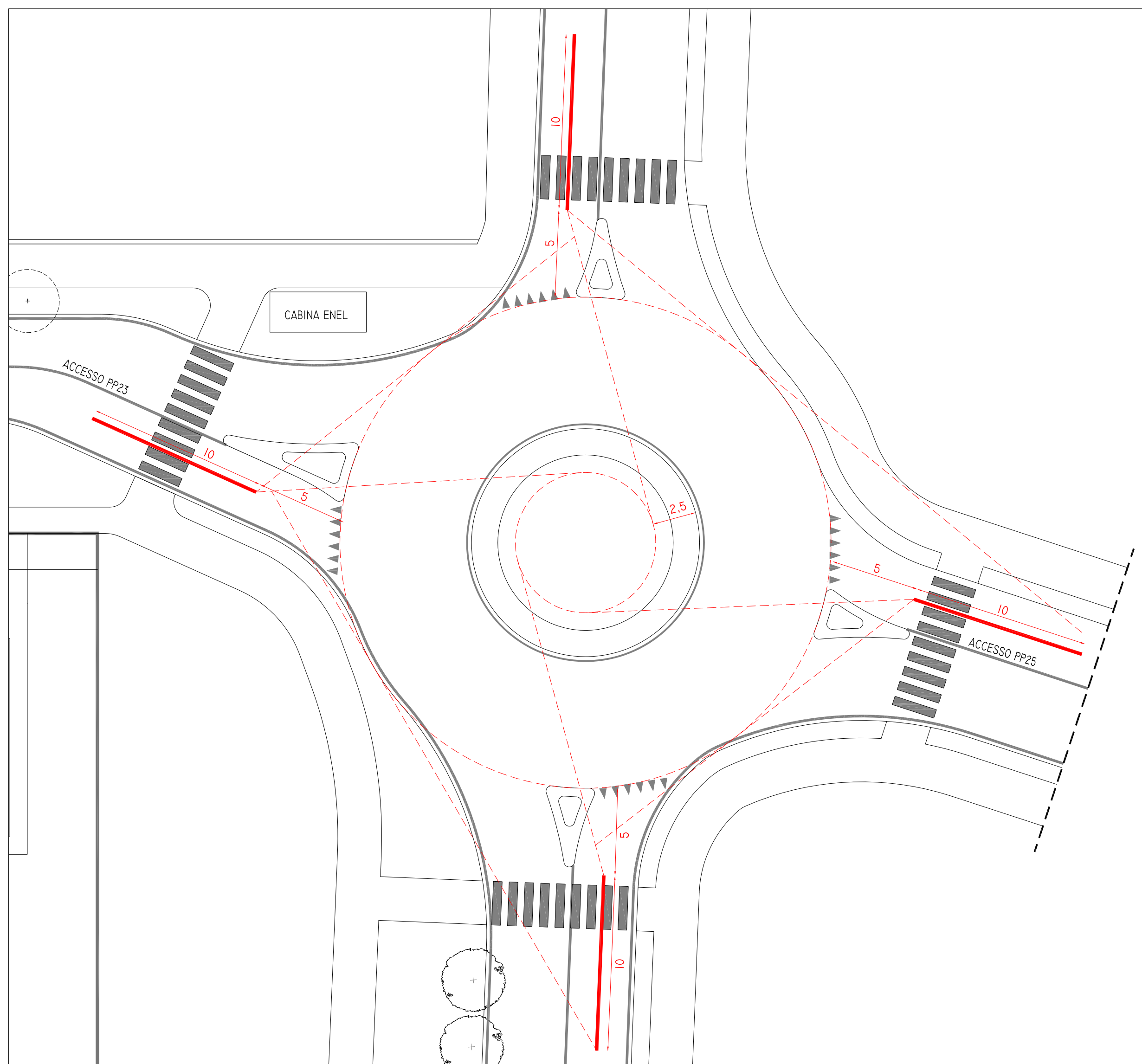
PLANIMETRIA SCALA 1:200 ⊕ VERIFICA CAMPI DI VISIBILITA' - DM 19/04/2006
